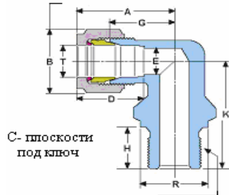
ШЕСТИГРАННИК ГАЙКИ
