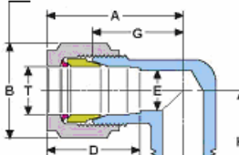
Р- ТРУБНАЯ РЕЗЬБА С- плоскости под ключ
