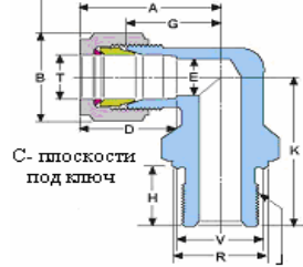
S- ЦИЛИНДРИЧЕСКАЯ РЕЗЬБА
