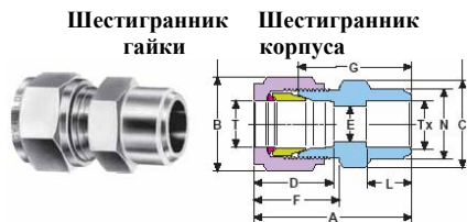
Сварочная трубная муфта: CW соединяет дюймовые трубы
